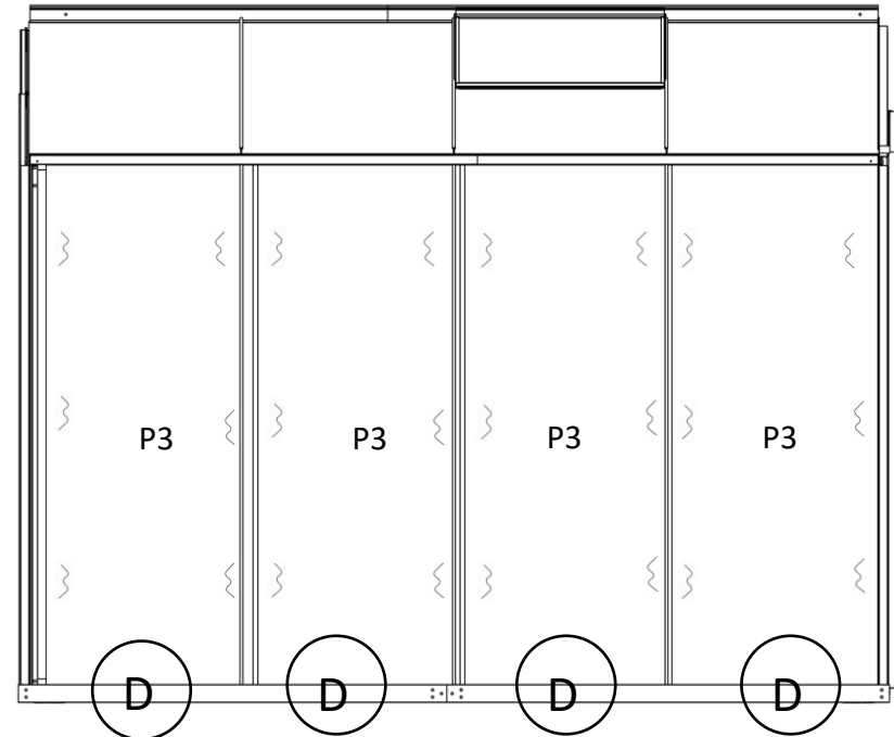
Pohled zepředu
