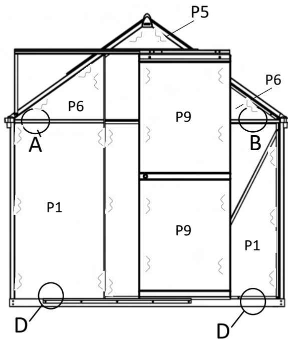
Čelní pohled
